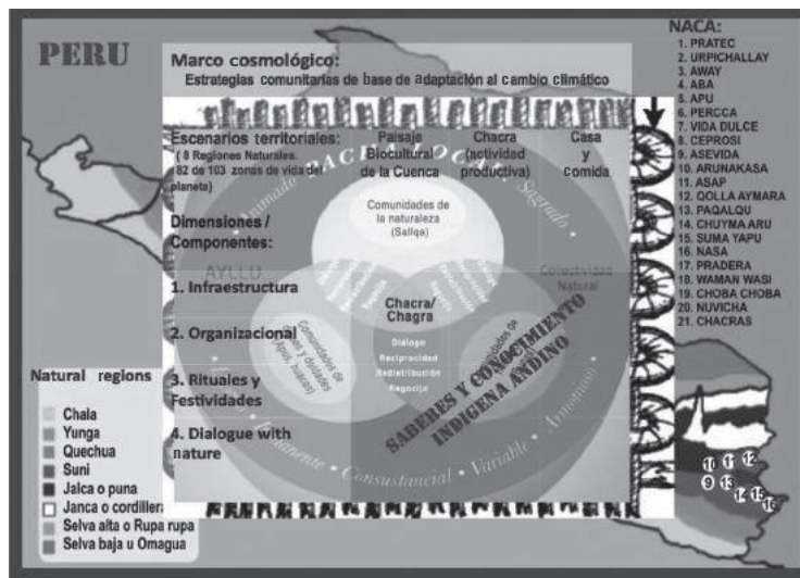
Figura 2. Marco cosmológico
